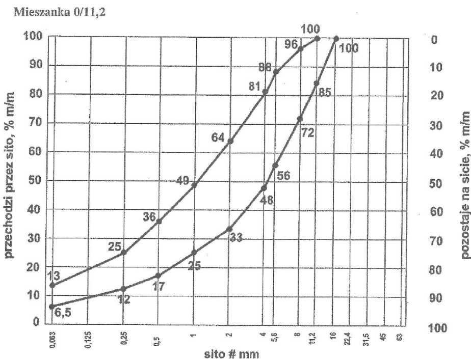
Rys.4. Uziarnienie mieszanki CBGM 0/11,2
