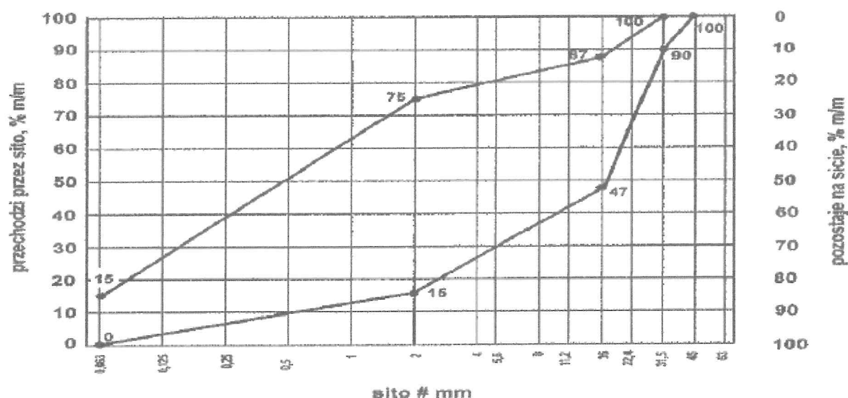
Rys. 2. Mieszanka niezwiązana 0/31,5 do nawierzchni z kruszywa niezwiązanego
