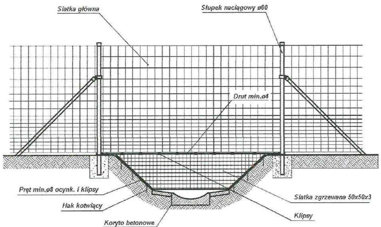
11.2.2. Zabezpieczenie ogrodzenia nad rowem w postaci siatki stalowej zgrzewanej o oczkach 50 \times 50 mm, przymocowanej nieruchomo w zagłębieniu rowu
