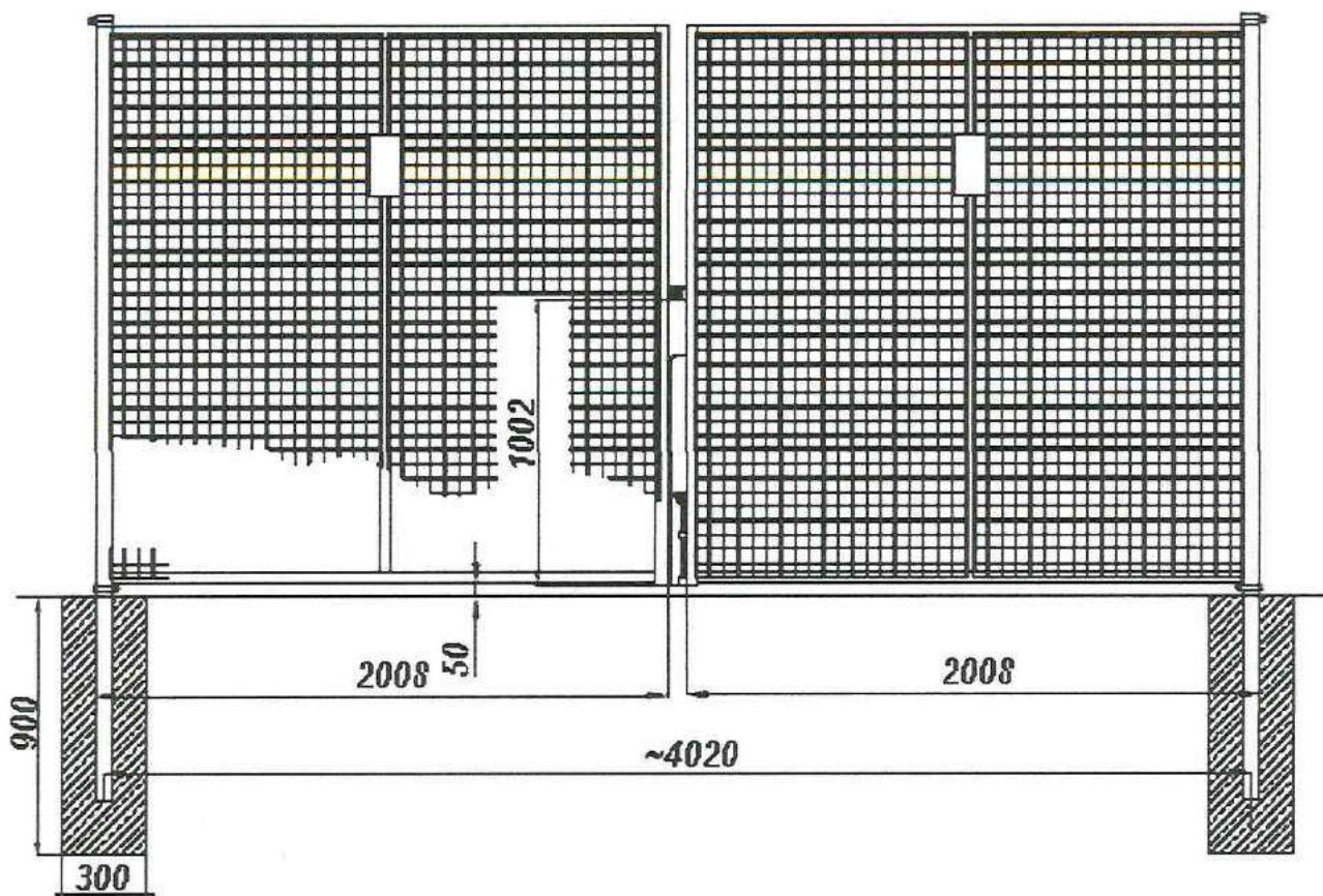
b) Furka szerokości 1 m
