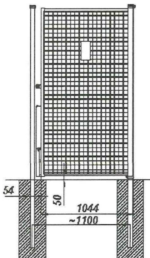
b) Furka szerokości 1 m
