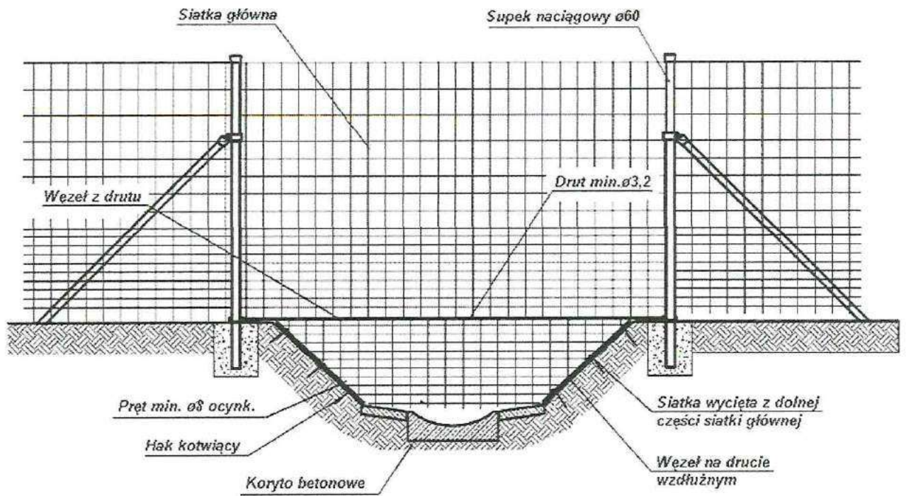
11.2.2. Zabezpieczenie ogrodzenia nad rowem w postaci siatki stalowej zgrzewanej o oczkach 50 \times 50 mm, przymocowanej nieruchomo w zagłębieniu rowu
