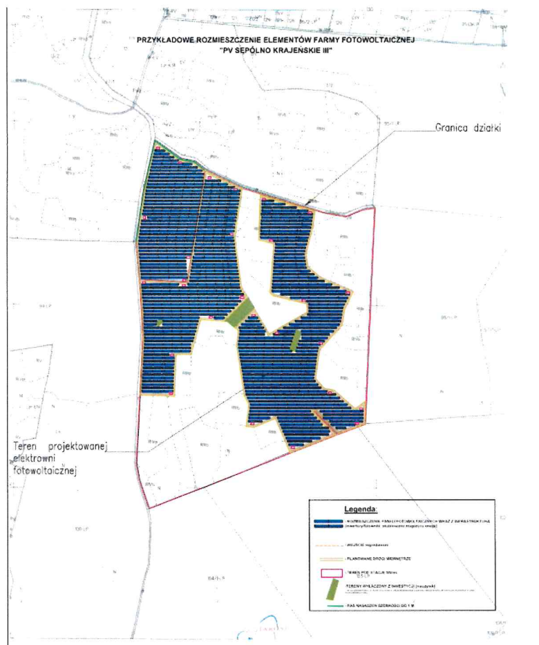
Rozmieszczenie elementów instalacji oraz planowanych nasadzeń (linia zielona - pogrubiona) zgodnie z planem zawartym w uzupełnieniu raportu z dnia 16 września 2022 r.
