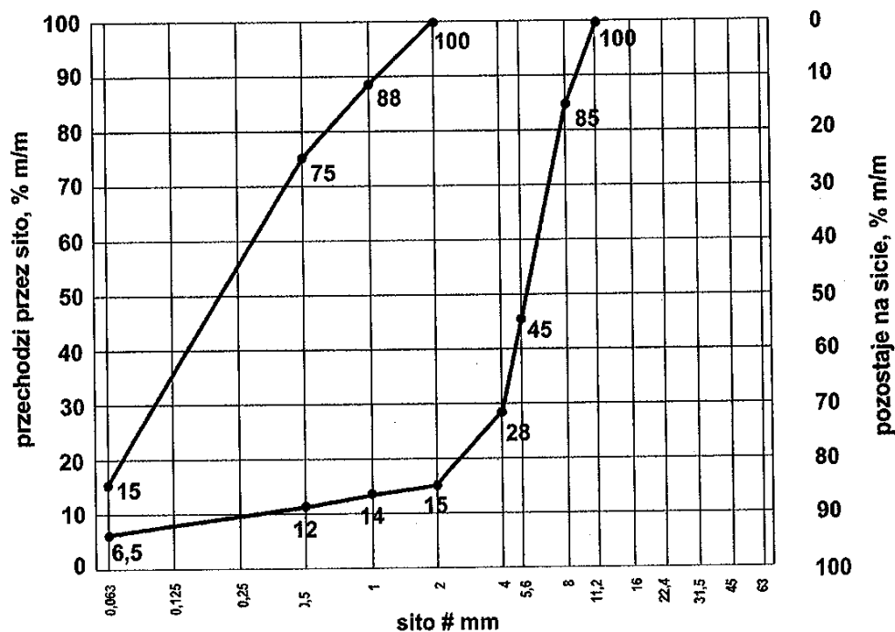
Rys.5. Uziarnienie mieszanki CBGM 0/8
