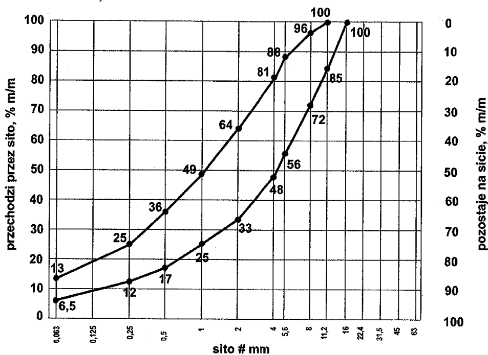
Rys.4. Uziarnienie mieszanki CBGM 0/11,2
