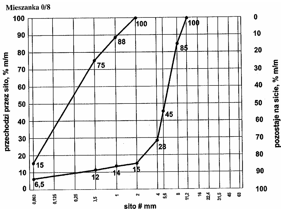
Rys.5. Uziarnienie mieszanki CBGM 0/8
